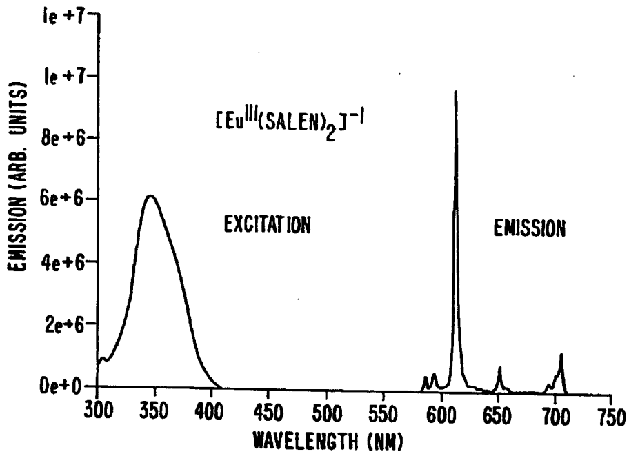
FIG. 23B.
